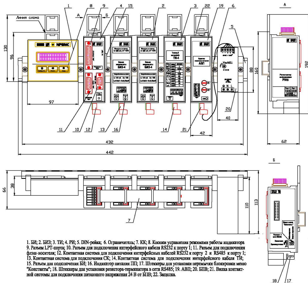
Габаритные и присоединительные размеры БВП ИРВИС-РС4* (бескорпусное исполнение)
