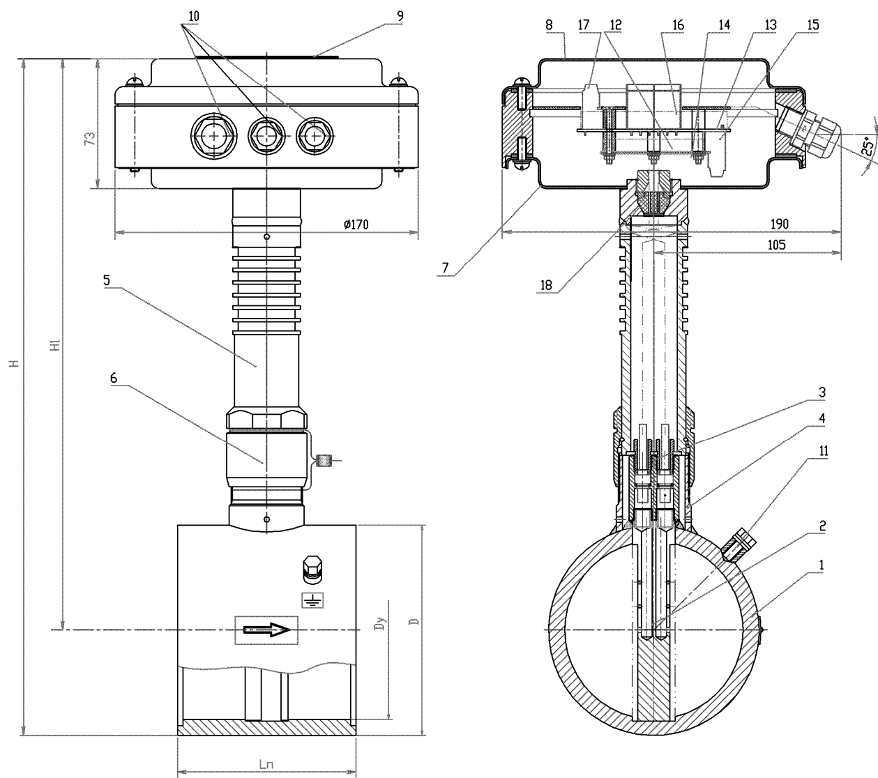
Конструкция, габаритные и присоединительные размеры ППР ИРВИС-РС4-Пар
