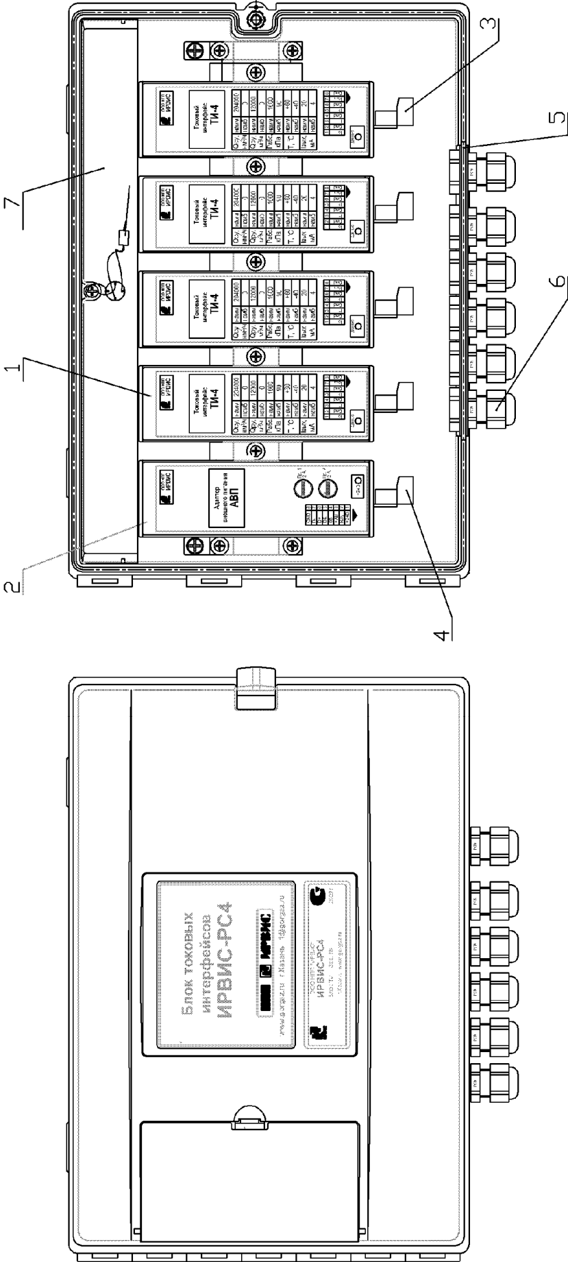
Вид при снятой крышке корпуса
